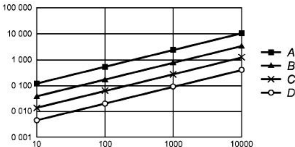
Рисунок А.3 - Классы герметичности (см. EN 1507 [5] и EN 12237)
