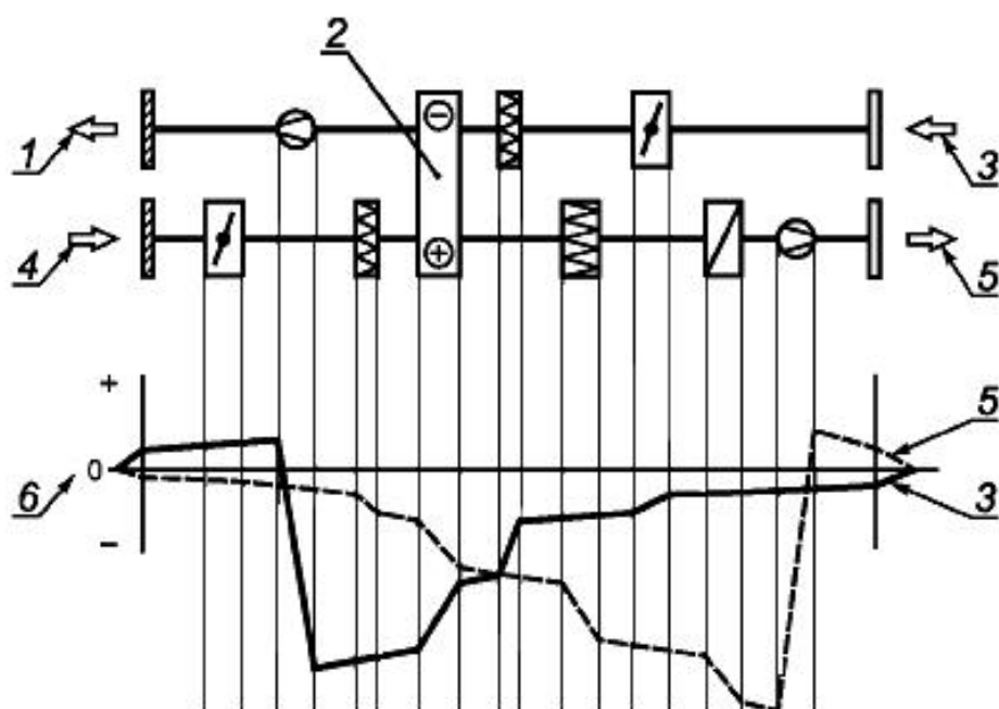
Рисунок А.2 - Перепады давления в системе
