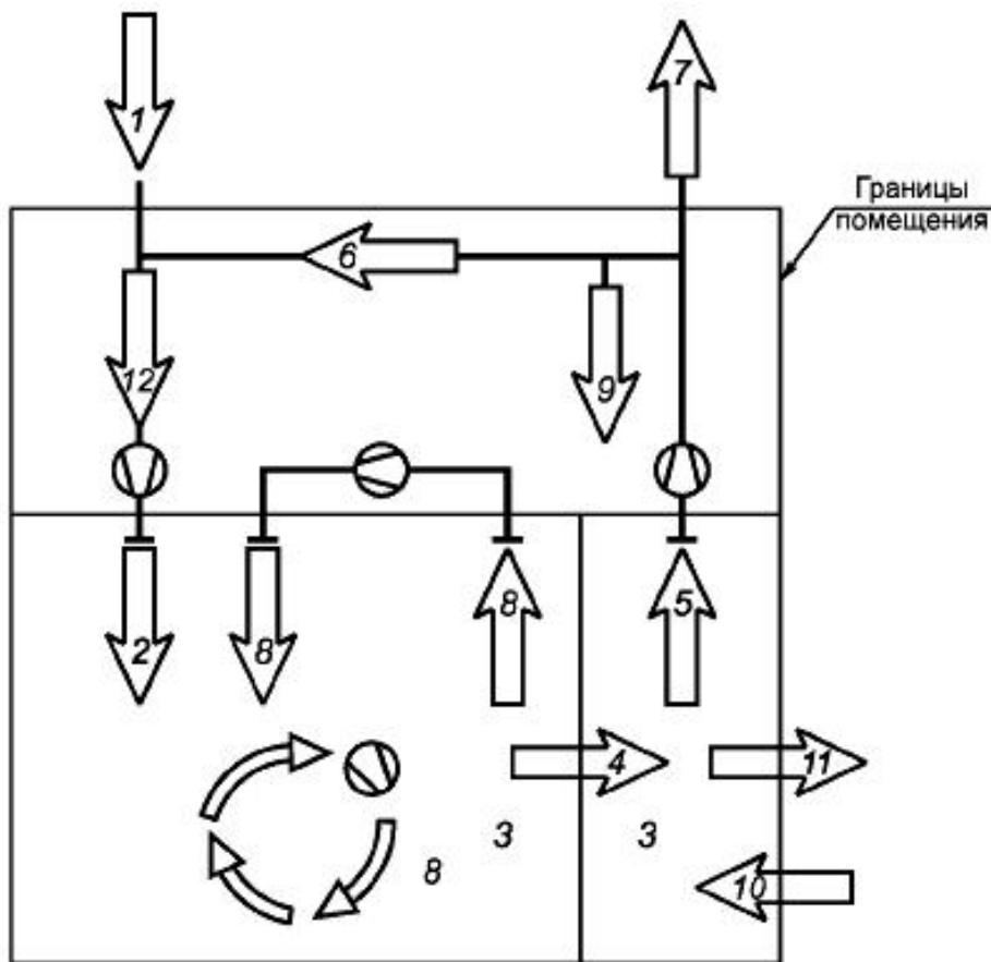
Рисунок 1 - Типы потоков воздуха. Номера позиций соответствуют таблице 2
